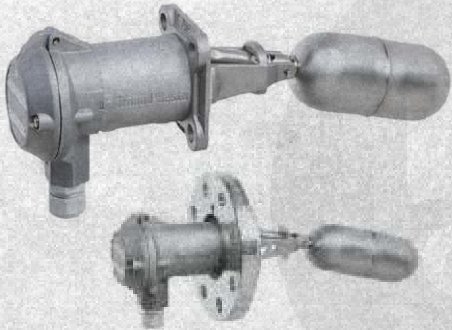
• Transmisor de nivel neumático
